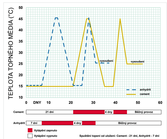
Příklad náběhového diagramu podlahového topení
